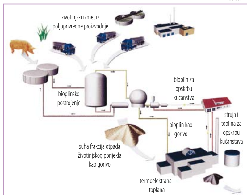
Ilustracija 10 Bioplinsko postrojenje kao dio energetskog sustava
