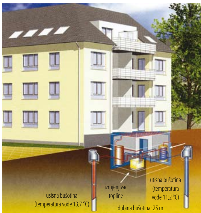
Ilustracija 12 Shema dizalica topline voda - voda u naselju Niehler WohnArt u Kölnu
